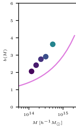
sim bias v fake mass est.
