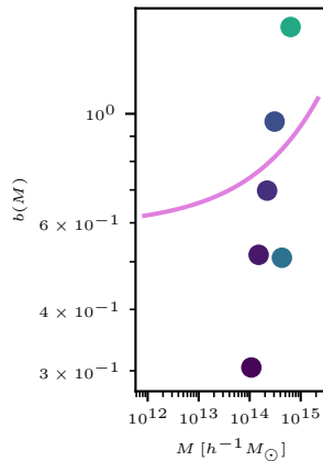
sim bias v fake mass est.
