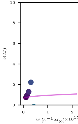
sim bias v fake mass est.
