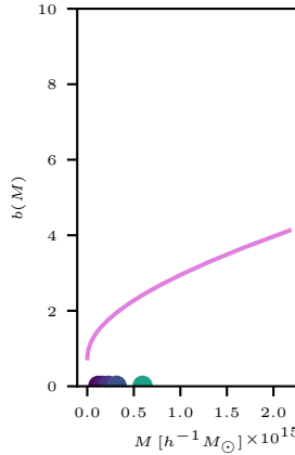
sim bias v fake mass est.
